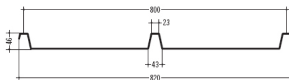
20 UNIMETAL 46 400 / 46
