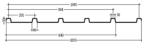
04 PORTA SIDERURGICA 201 / 30
