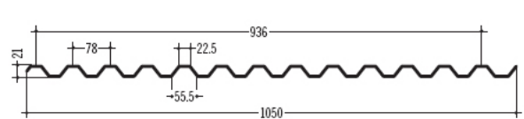
69 ALUBEL 21 78 / 22.5
