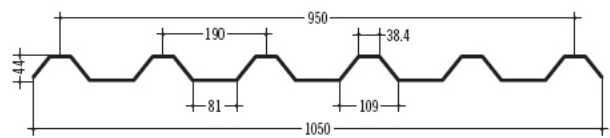
34 UNIMETAL 45 190 / 45
