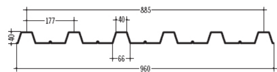
118 SOLIDLUX PERFIL 01 177 / 40
