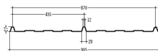
146 UNIMETAL G2007 435 / 27
