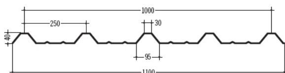
107 ASPERSA PERFIL 40/250 250 / 40
