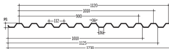
110 CENTROMETAL SILMA 28 112 / 28
