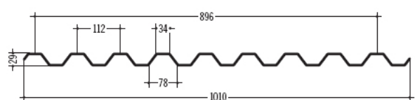
63 COPERNIT COPERALL 29 112 / 29
