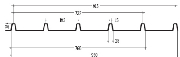
05 BROLLO EGB 401 183 / 38
