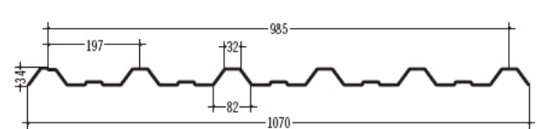
59 CENTROMETAL SILMA 6 197 / 34
