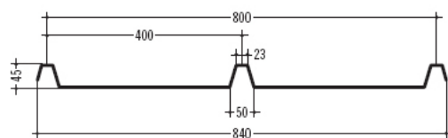
06 SAIP 45/800 400 / 45
