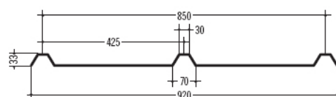
14 E.I.P. H32-G3-P850 425 / 33
