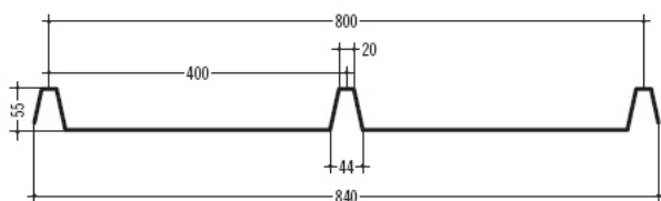
17 BROLLO EGB 700 400 / 55
