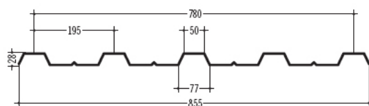
122 ACERALUM 02 195 / 28
