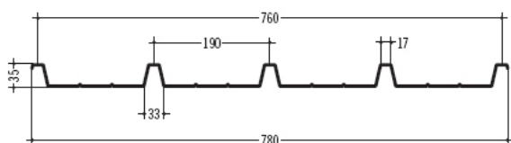
13 ZANOLETTI CTZ 760 190 / 35
