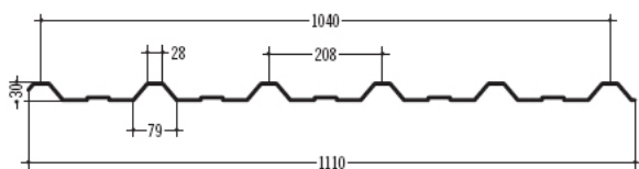
129 PERCASA PC-30 208 / 30
