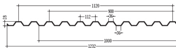
137 EDILFIBRO METAPLAK 28 112 / 28
