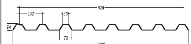
60 CENTROMETAL SILMA 8 132 / 32
