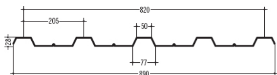
121 ACERALUM 01 205 / 28
