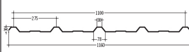
88 TECZONE TZ - 30 275 / 30
