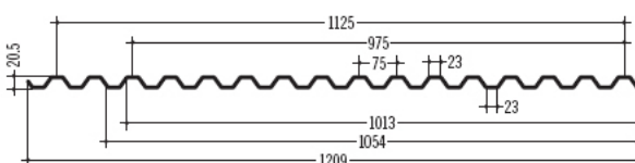
117 MARANIT METALPLUS 20 75 / 20
